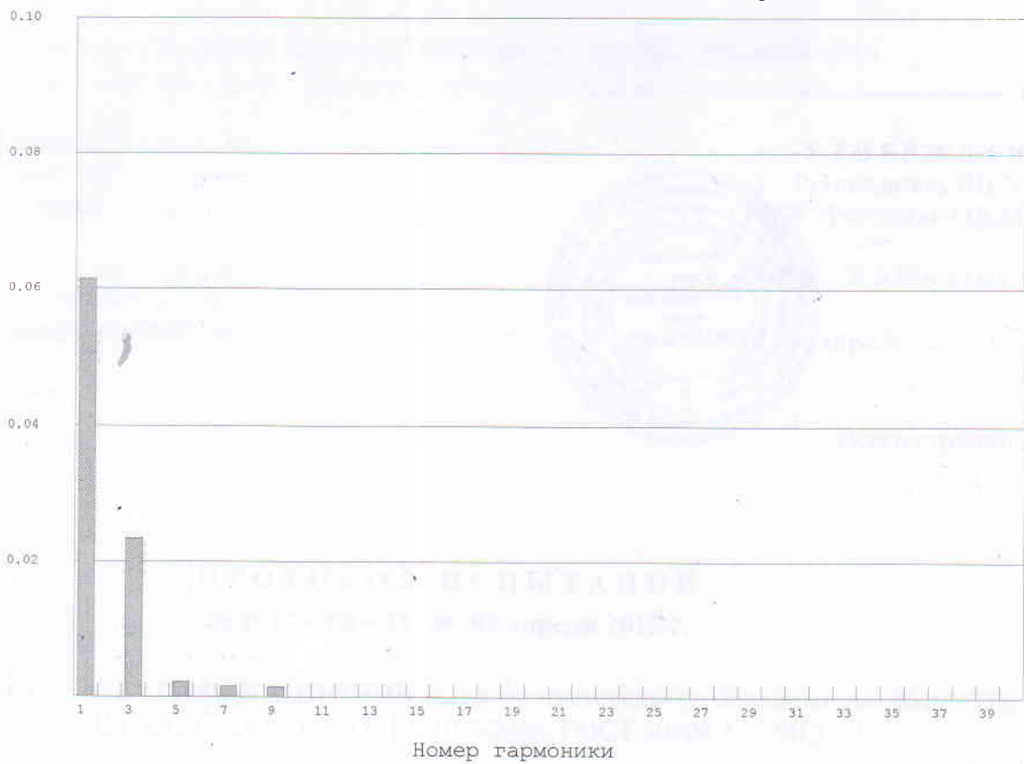
Эмиссия гармонических составляющих тока (усредненная)
